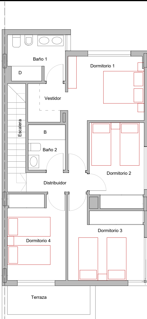
Planta alta
