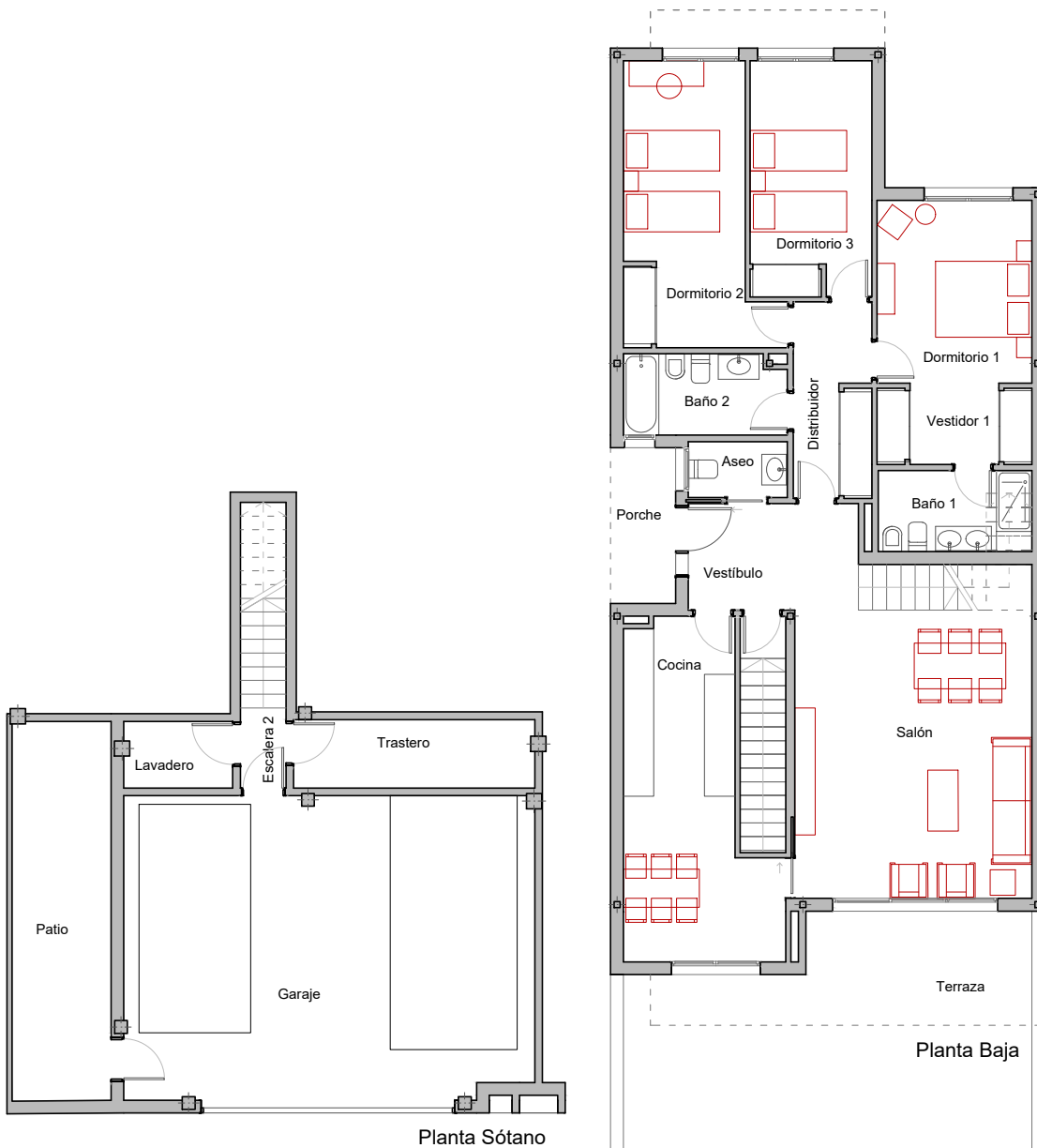
Planta Sótano
